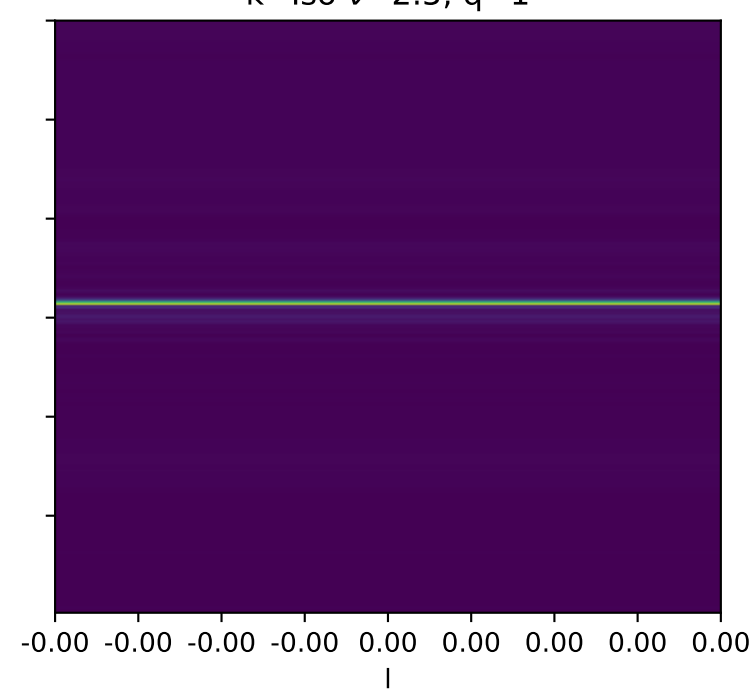
k=Iso \nu=2.5 , q=1
