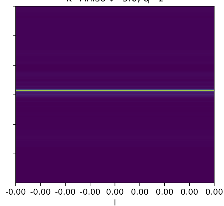
k=Aniso \nu=3.0 , q=1
