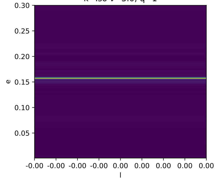
k=Iso \nu=3.0 , q=1
